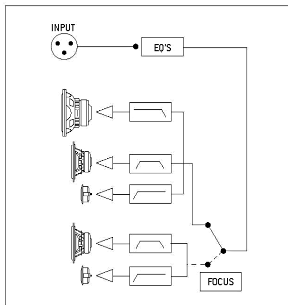
Diagrama de modo FOCUS de los monitores TRI06 Be.
