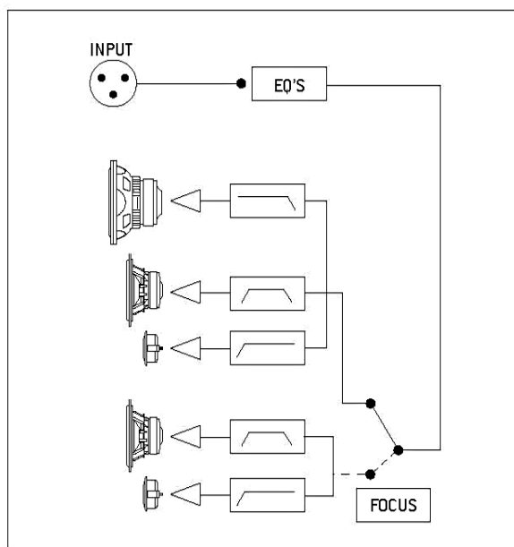
TRIO6 Be FOCUS 模式图标.
