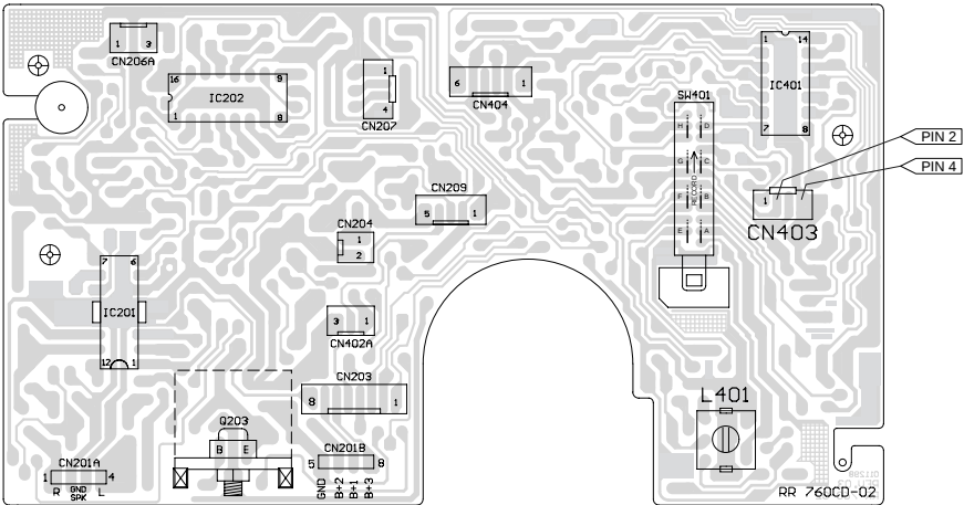
Verstärkerplatte
