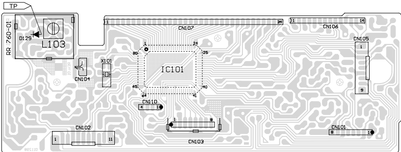
CPU-Platte
