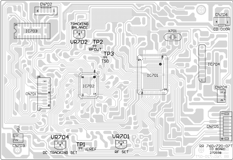
CD-Servo-Platte
