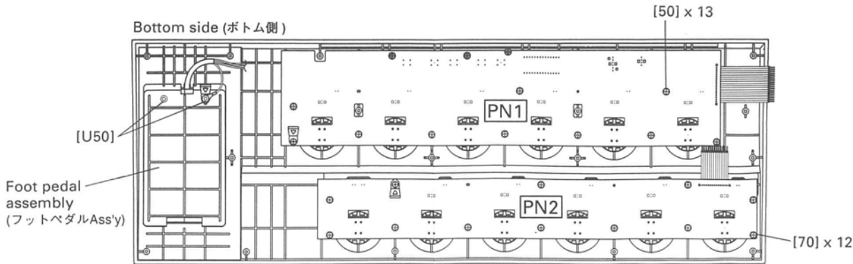
[50]:Bind Head Tapping Screw-B 3.0X8 MFZN2BL (EP600190) + バインド B タイト [70]:Bind Head Tapping Screw-B 3.0X8 MFZN2BL (EP600190) + バインド B タイト [U50]:Bind Head Screw SP 3.0X12 MFZN2Y (VB763800) + バインド小ネジ
