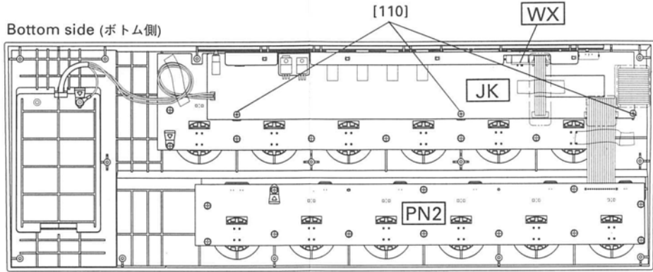
[110]:Bind Head Tapping Screw-B 3.0X8 MFZN2BL (EP600190) + バインド B タイト (Fig. 3)
